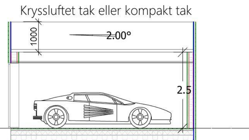
Snitt C-C
