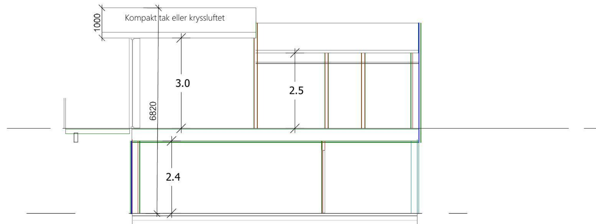
Snitt B-B
